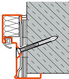
Diagonalbefestigung (Sichtmauerwerk / Beton)
