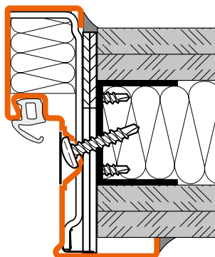
Diagonalbefestigung (Metallständerwand mit Aussteifungsprofil lt. statischer Erfordernis). Bei dieser Montageart ist die Montage nur mit Türschließer zulässig!
